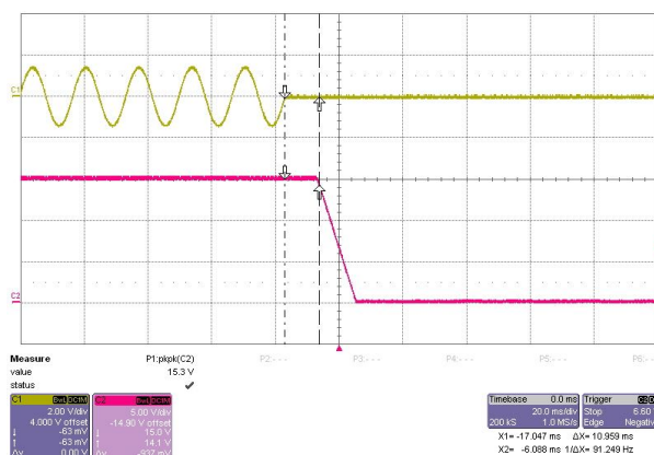
FS10-15 11.0mS
