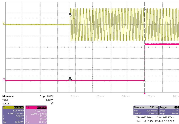
FS10-3R3 0.85S
