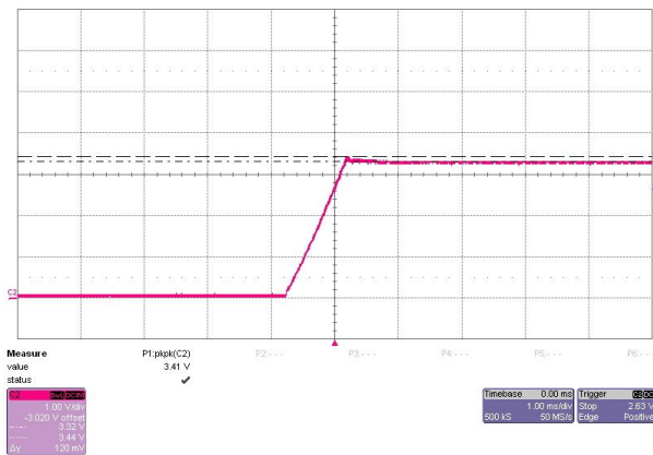
FS10-3R3 0.12V
