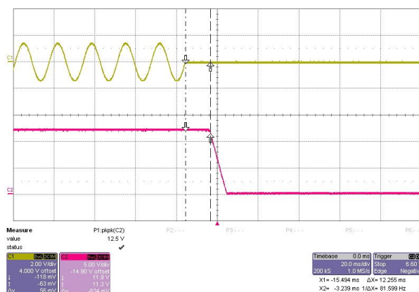
FS10-12 12.3mS
