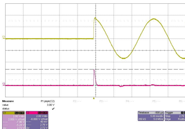
FS10-24 13.6A
