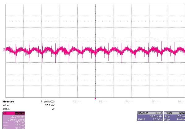
FS10-24 37.6mVpp
