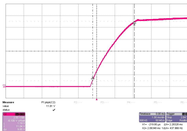
FS10-12 2.83mS
