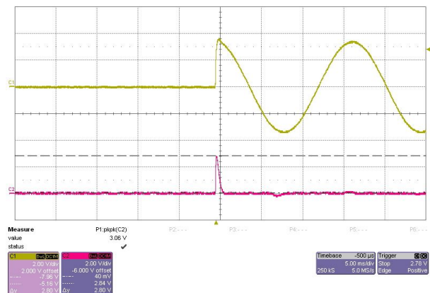
FS10-15 14.0A
