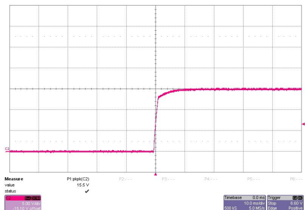
FS10-15 0V
