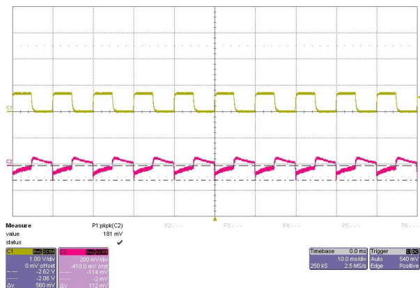
FS10-15 112mV
