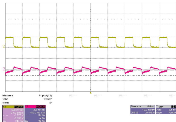
FS10-24 96mV
