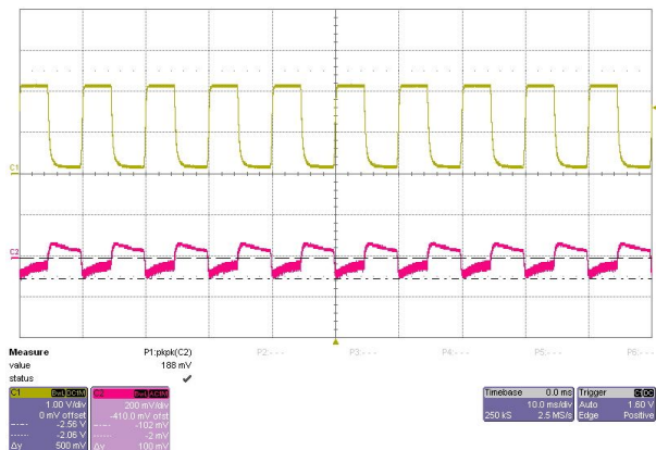
FS10-5 100mV
